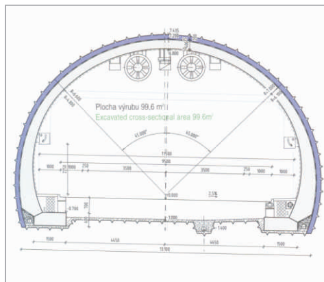
Vzorový příčný řez raženého tunelu.
